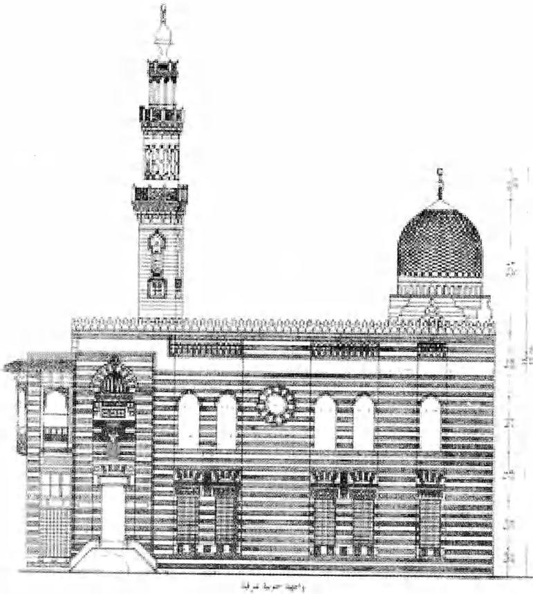
شكل رقم (١٢): مدرسة الأشرف برسباي - الواجهة الجنوبية الشرقية.
